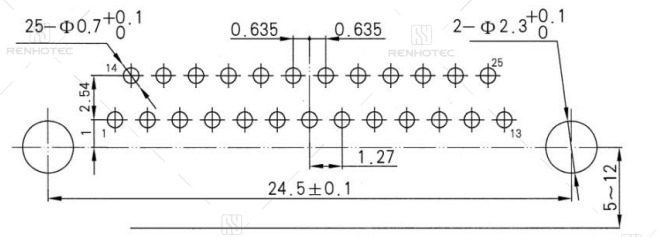
J30J-25ZKW-J
