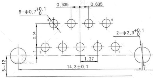
J30J-9TJW-J
