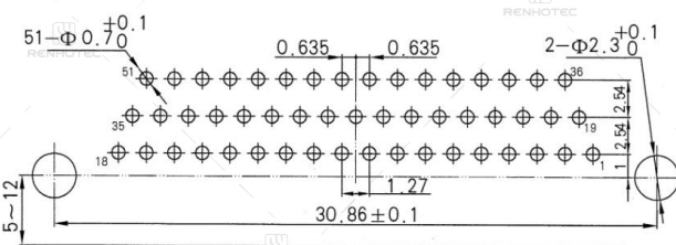
J30J-51TJW-J
