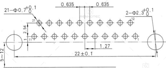
J30J-21TJW-J
