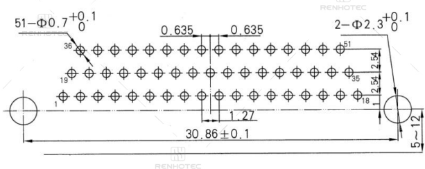
J30J-51ZKW-J
