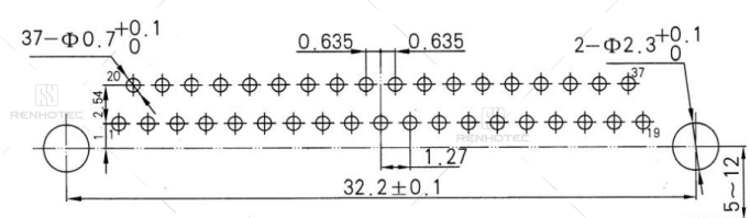
J30J-37ZKW-J
