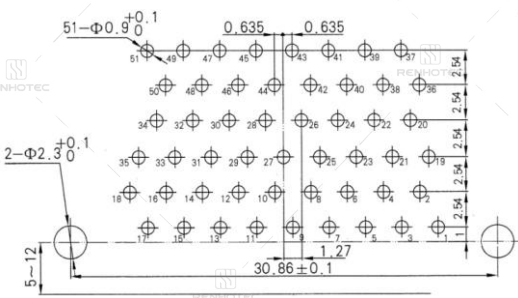
J30J-51TJW
