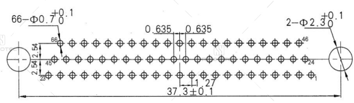
J30J-66TJN-J
