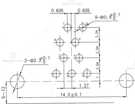
J30J-9ZKW
