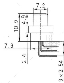
J30J-51, 66ZKW-J
