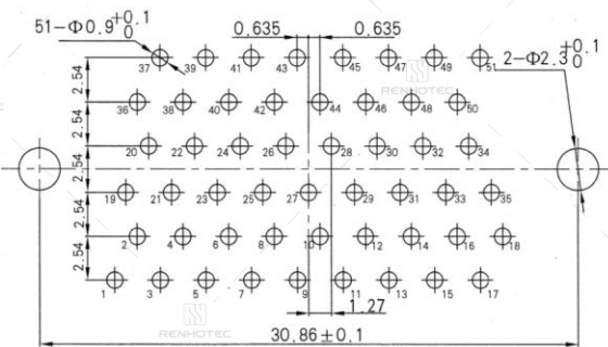
J30J-51ZKN
