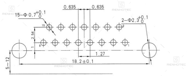
J30J-15TJW-J
