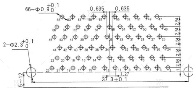
J30J-66TJW
