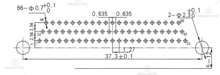
J30J-66ZKW-J
