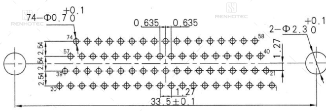
J30J-74TJN-J
