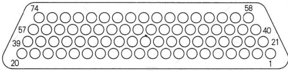
J30J-74
