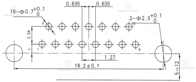
J30J-15ZKW-J
