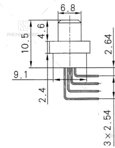
J30J-74, 100TJW-J
