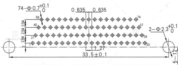
J30J-74ZKW-J
