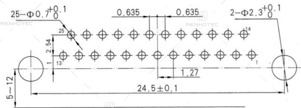
J30J-25TJW-J
