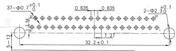
J30J-37TJW-J
