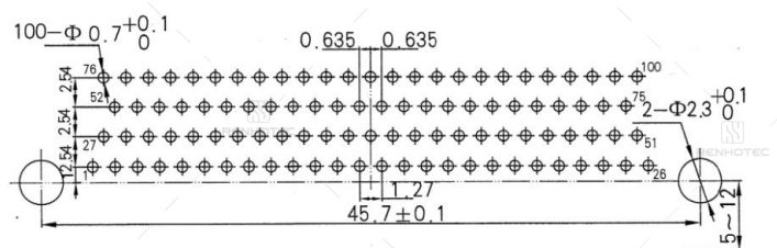
J30J-100ZKW-J
