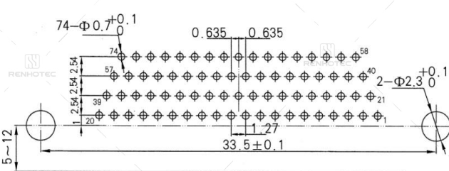
J30J-74TJW-J
