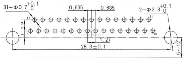
J30J-31ZKW-J
