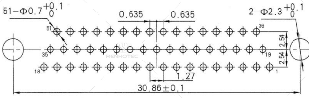
J30J-51TJN-J
