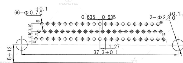
J30J-66TJW-J
