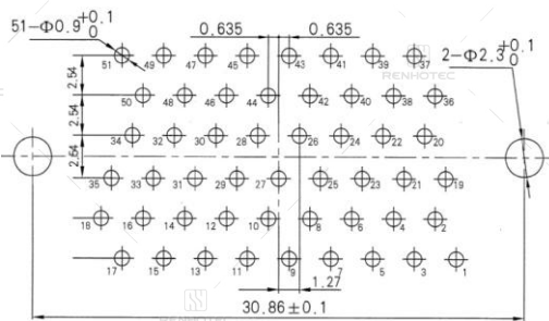
J30J-51TJN
