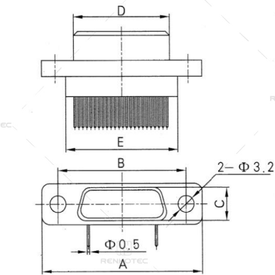
J30J-9~100ZKW-J
