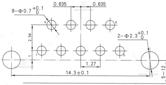
J30J-9ZKW-J
