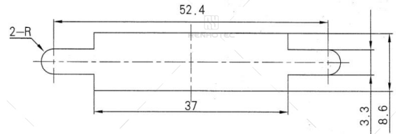
J30J-100TJ-Q/ZK-Q
