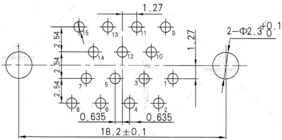
J30J-9TJN
