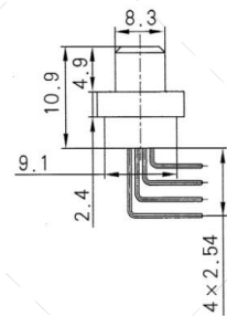
J30J-74, 100ZKW-J
