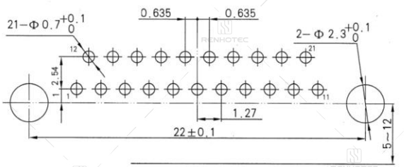
J30J-21ZKW-J
