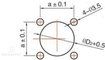
安装开口尺寸：Mounting Dimensions
