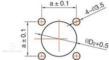
安装开口尺寸: Mounting Dimensions
