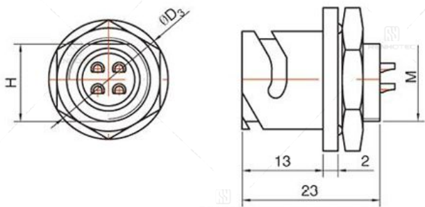
圆盘插座 Circular Receptacle:
