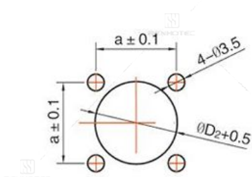
安装开口尺寸：Mounting Dimensions
