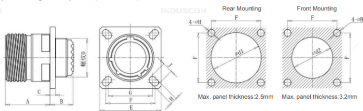
Square Flange Receptacle (D38999/20)
