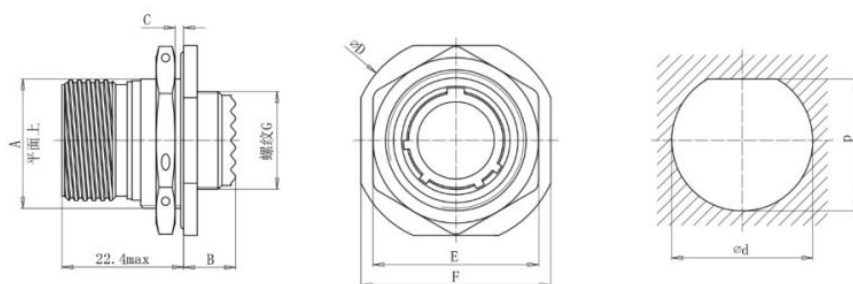
Jam Nut Receptacle (D38999/24)
