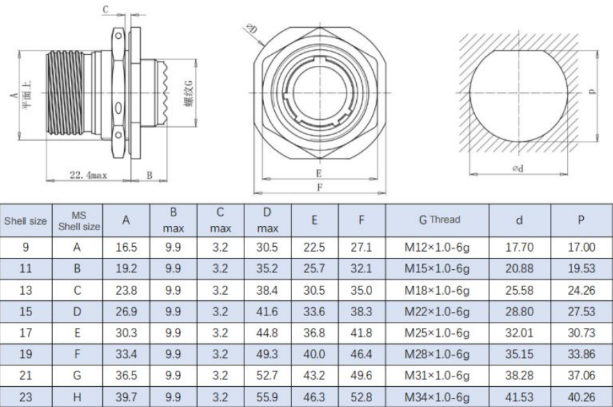
Jam Nut Receptacle (D38999/24)
