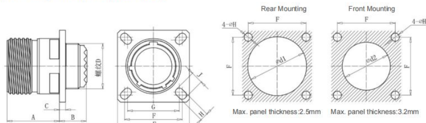
Square Flange Receptacle (D38999/20)
