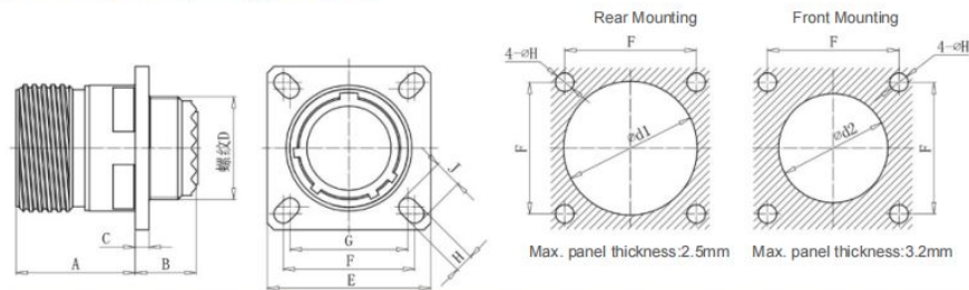
Square Flange Receptacle (D38999/20)
