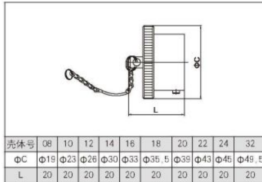
【80插头金属防尘盖】
