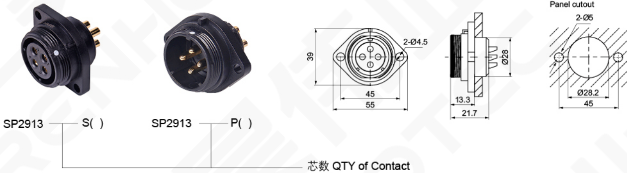
2 孔法兰插座 SP2913 系列 2-hole flange SP2913 Series
