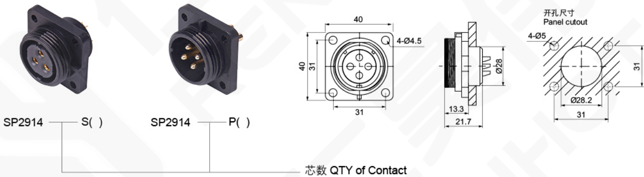
4 孔方形插座 SP2914 系列 4-hole Square SP2914 Series
