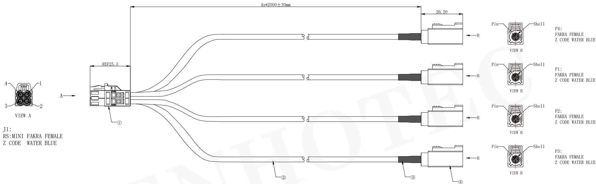
Wiring Table
