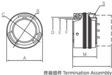
终端组件 Termination Assembly
