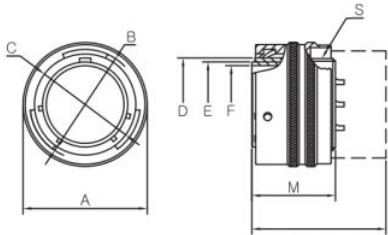
终端组件 Termination Assembly
