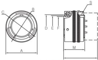
终端组件 Termination Assembly
