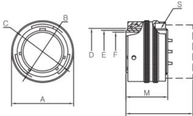
终端组件 Termination Assembly
