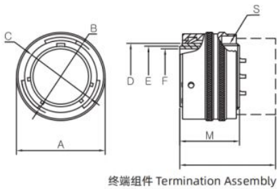
终端组件 Termination Assembly
